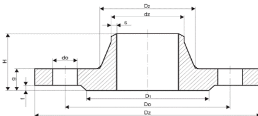
Kolnierz z szyjką wg DIN 2633
